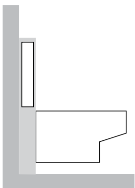
Soluție cu vas WC suspendat
